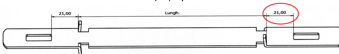
distanziatore AM/21 per pannelli da 21mm.
