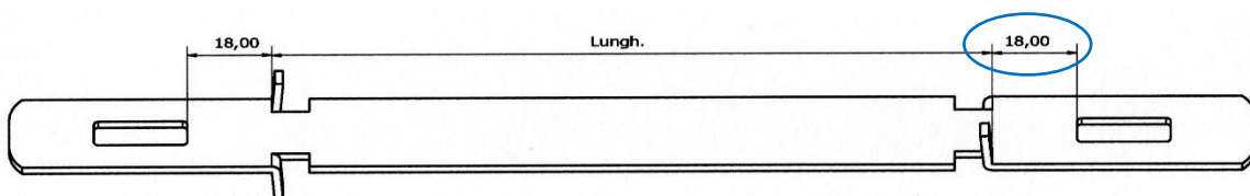
distanziatore AM/18 per pannelli da 18mm.
